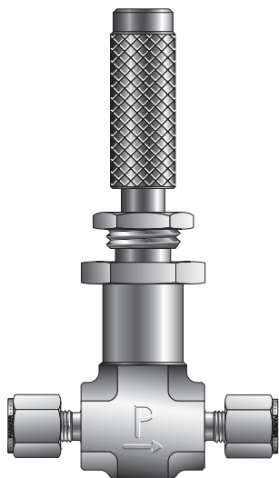
Model Shown: 2A-NML-V-SS-K
