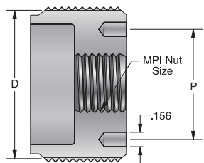
Figure 56: MPI™ Nut Die
